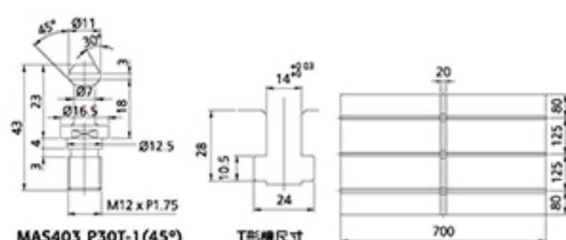
MAS403 P30T-1(45°)
